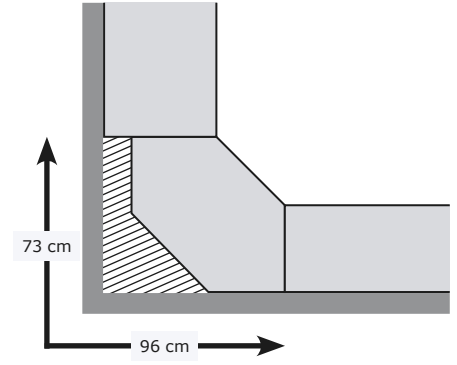
35 cm derinliğinde bir iskelet ve 58 derinliğinde bir iskelet ile köşe bölümü.
